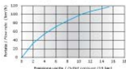
CURVA DI PORTATA / FLOW-RATE CURVE GAS: Aria / Air pressione ingresso / Inlet pressure 30 bar
