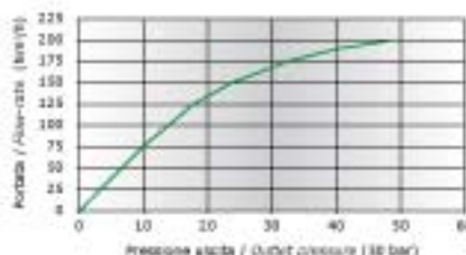
CURVA DI PORTATA / FLOW-RATE CURVE GAS: Aria / Air pressione ingresso / Inlet pressure 70 bar
